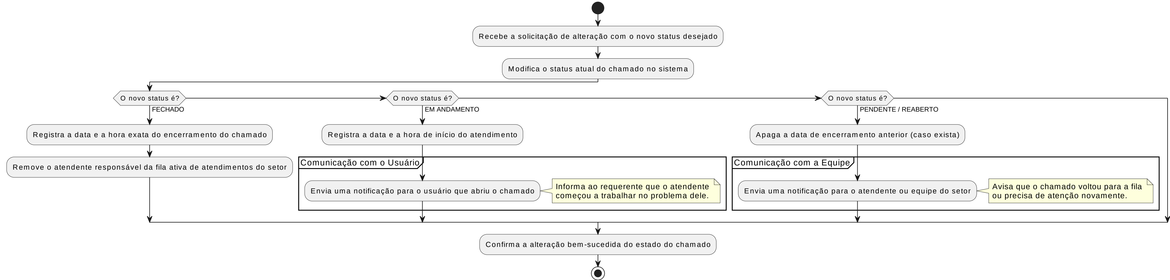
Diagrama de Atividade - Lógica de Alteração de Status do Chamado
